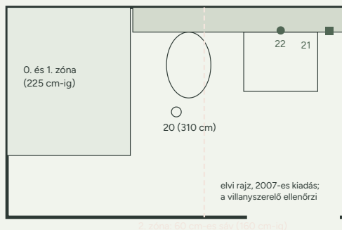
Elvi zónarajz a mintafürdőben, a szabvány 2007-es kiadásának összefoglalója szerint. A 3.4 lecke ábrája.
