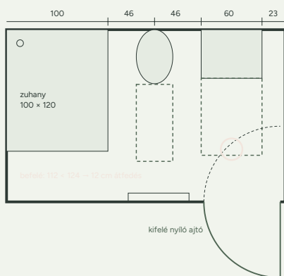
A mintafürdő kiosztása felülnézetben. A 2.2 lecke ábrája.
